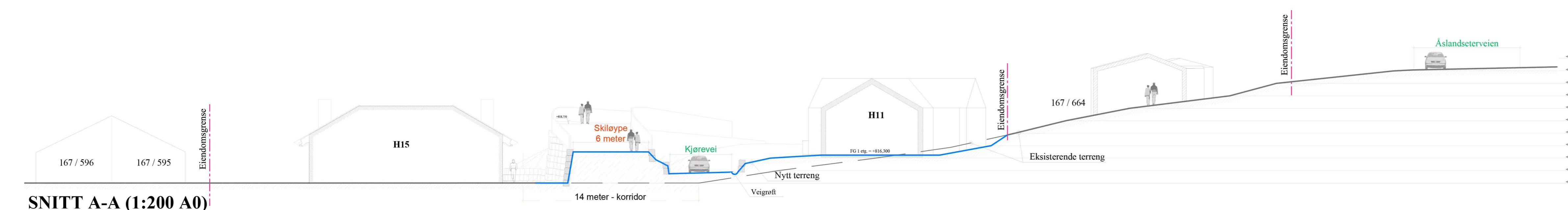
SNITT A-A (1:200 A0)
