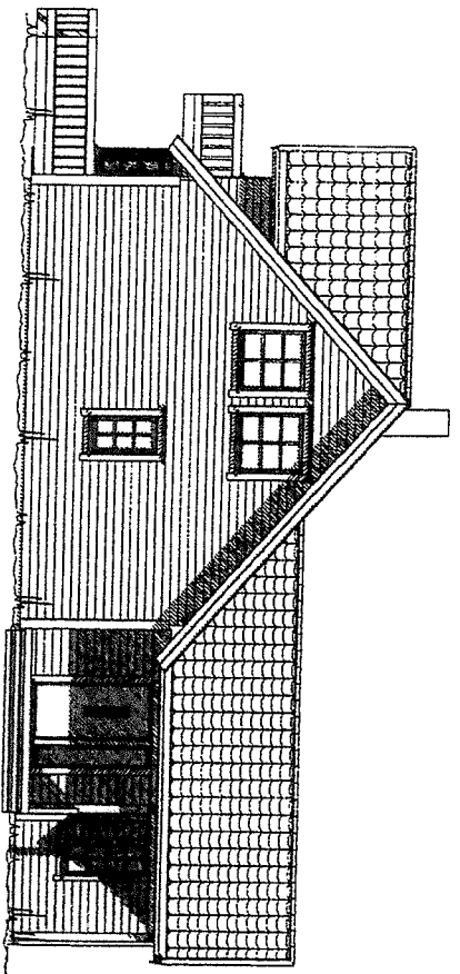
FASADE SØR
